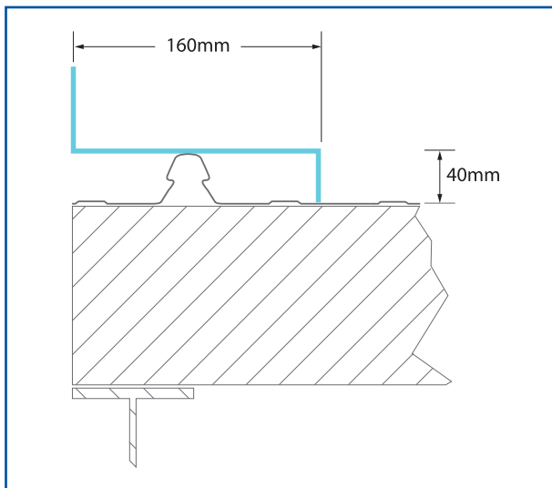
AU (Apron Uprand) - Metal Deck
